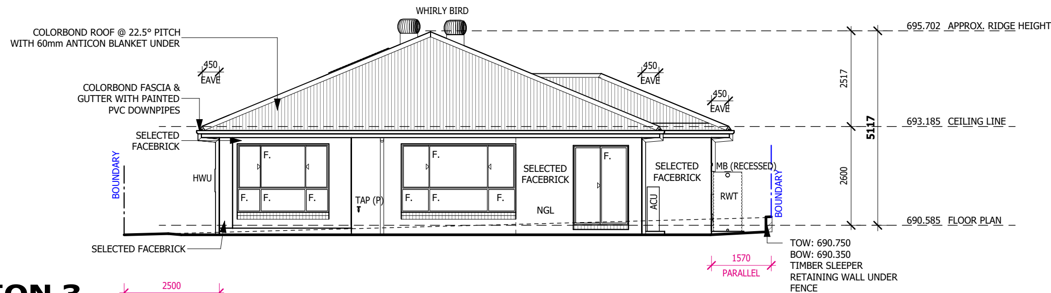
ELEVATION 3
