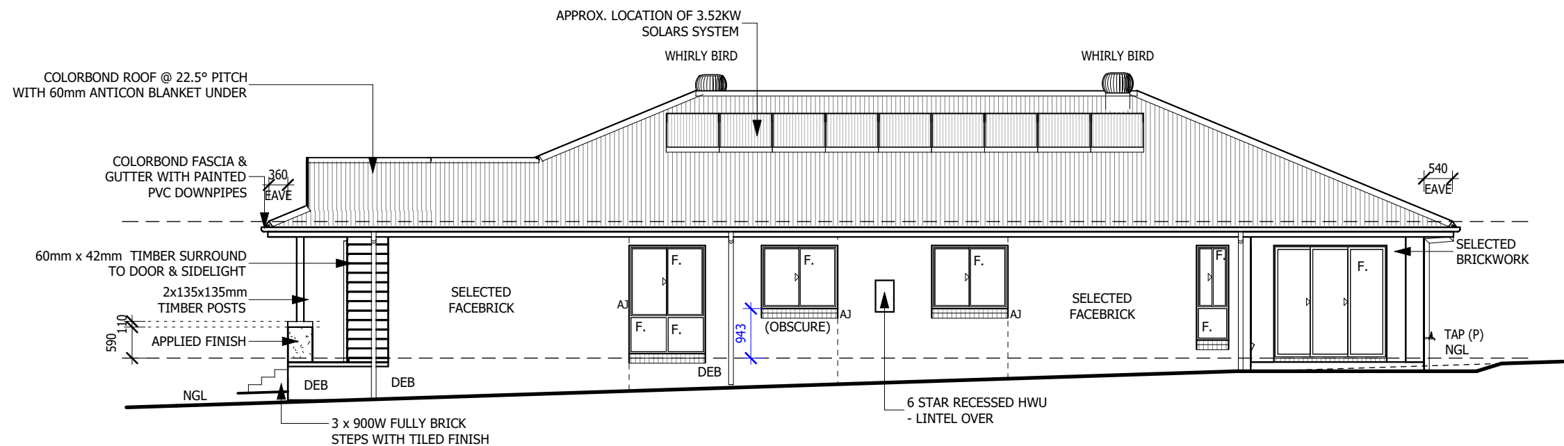
ELEVATION 2
